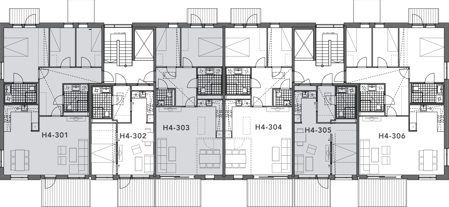
3. etasje
